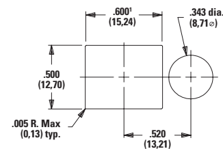
J52 Actuators
