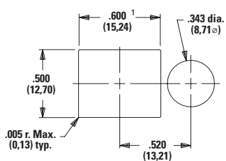
J62 Actuator
