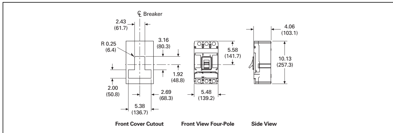
Figure 27.4-7. L-Frame
