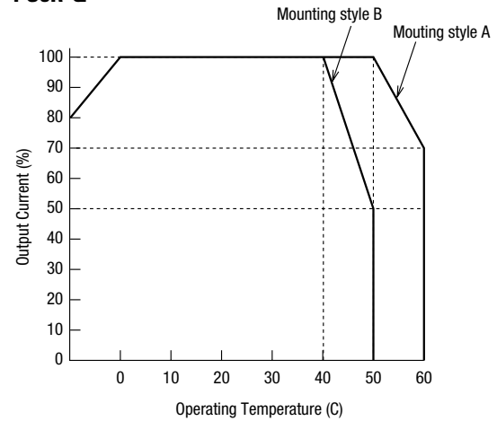
PS5R-Q
