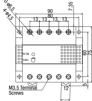
PS5R-D (50W)
