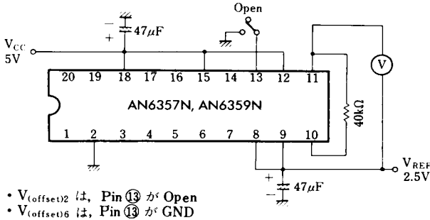
Test Circuit 8 (V O(offset)2 , V O(offset)6 )
