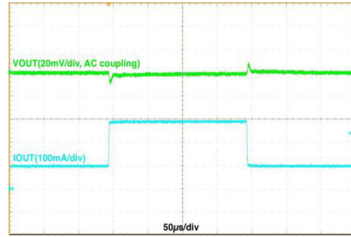
Figure 17. Load Transient, V_{IN} = 3.6\text{ V} , V_{OUT} = 1.8\text{ V} , 100\text{ mA} \leftrightarrow 300\text{ mA} , 1\text{ }\mu\text{s} Edge, Auto Mode
