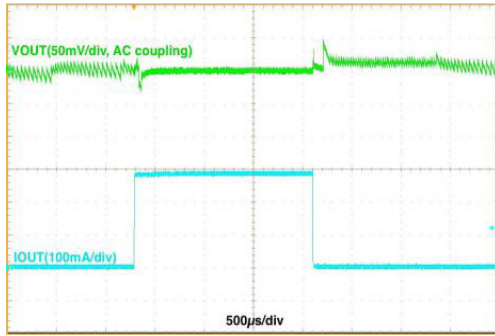
Figure 16. Load Transient, V_{IN} = 3.6\text{ V} , V_{OUT} = 1.8\text{ V} , 5\text{ mA} \leftrightarrow 300\text{ mA} , 1\text{ }\mu\text{s} Edge, Auto Mode
