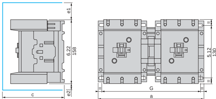
LC2D115 and D150 2 x LC1D115 and D150
