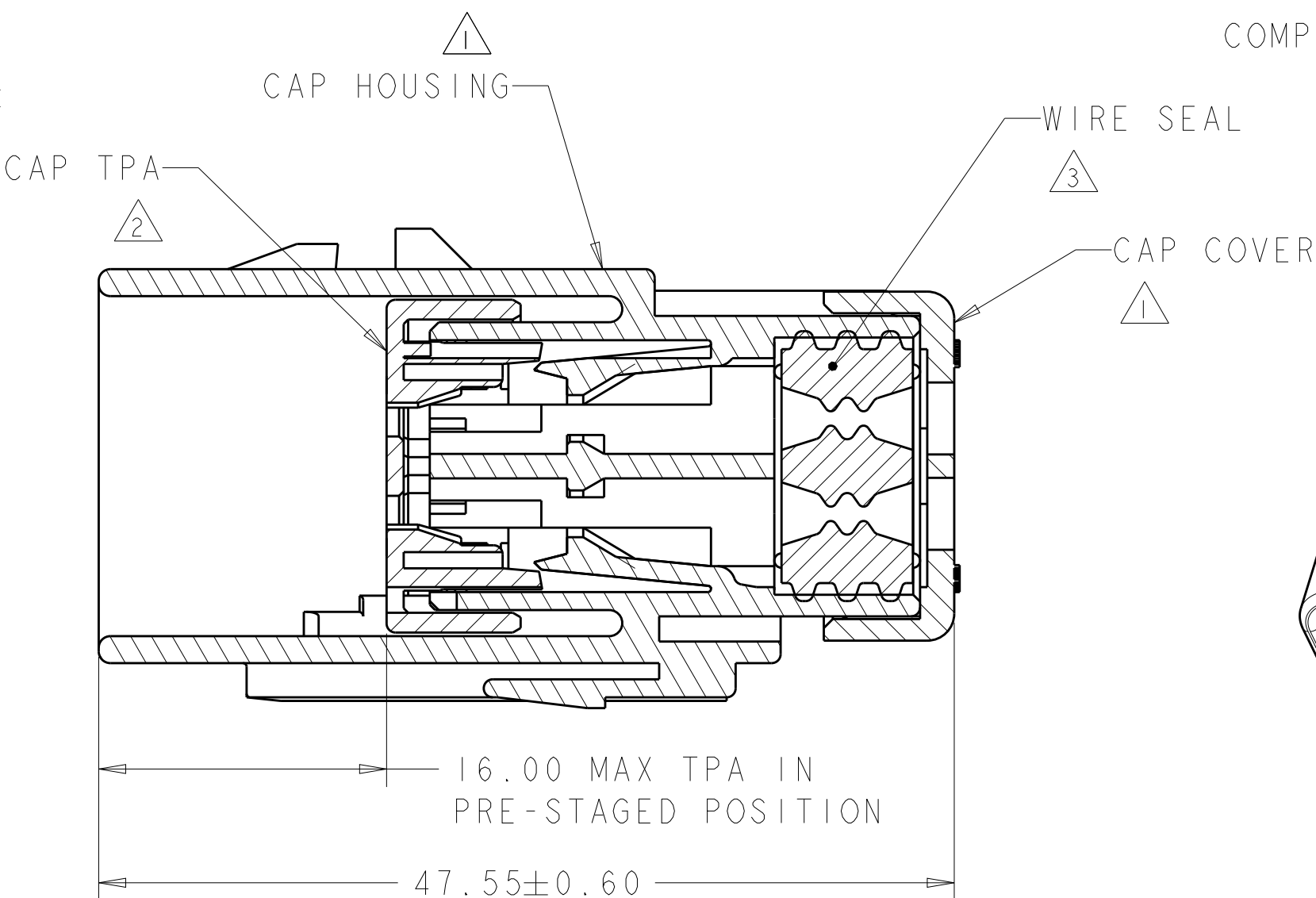
SECTION A-A
