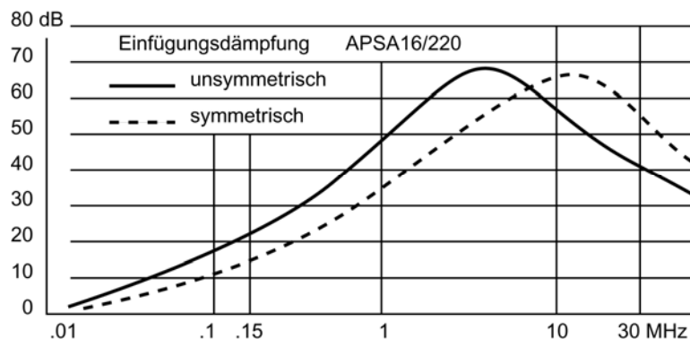
Fig. 2 Frequenzabhängige Dämpfung des EMV-Filters
