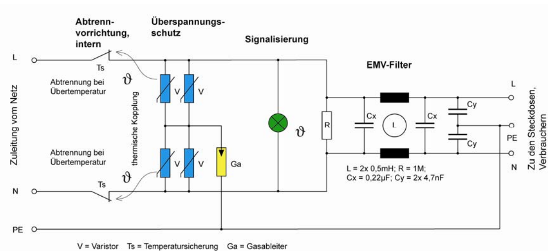
Fig. 1 Schaltbild Überspannungsschutz und EMV-Filter
