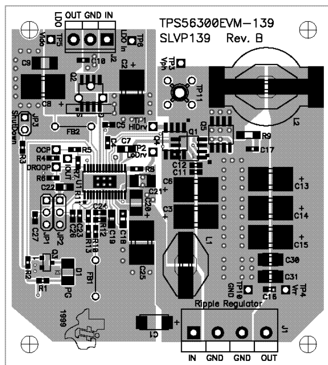
Figure 30. Top Layer
