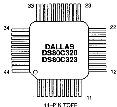
44-PIN TQFP
