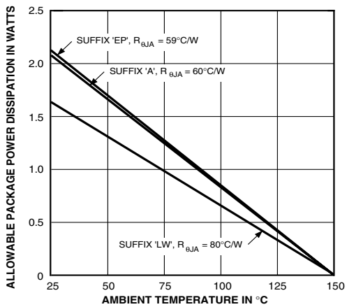
Dwg. GP-024B
