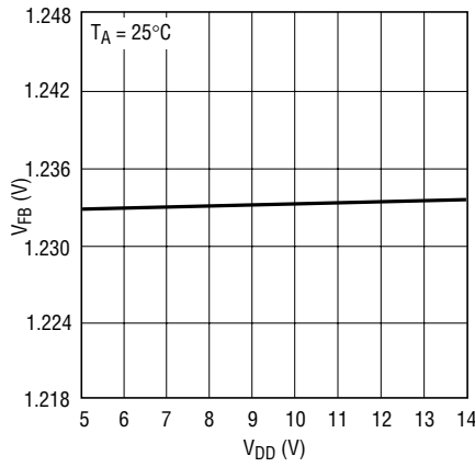
V FB vs V DD
