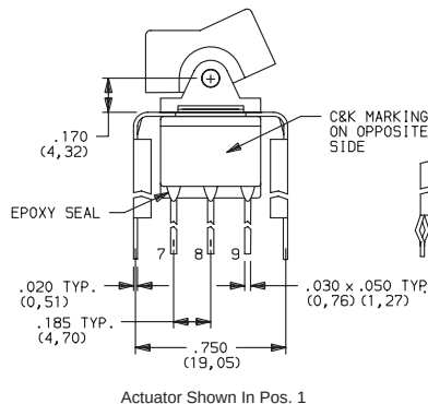
E301J1_BE2 3PDT
