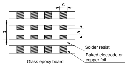
Fig.3 (in:mm)
