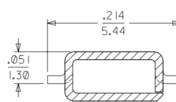
SECTION A-A 10:1
