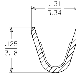
SECTION B-B 10:1
