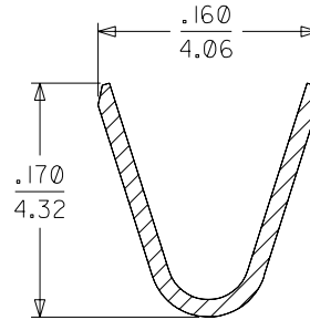
SECTION C-C 10:1
