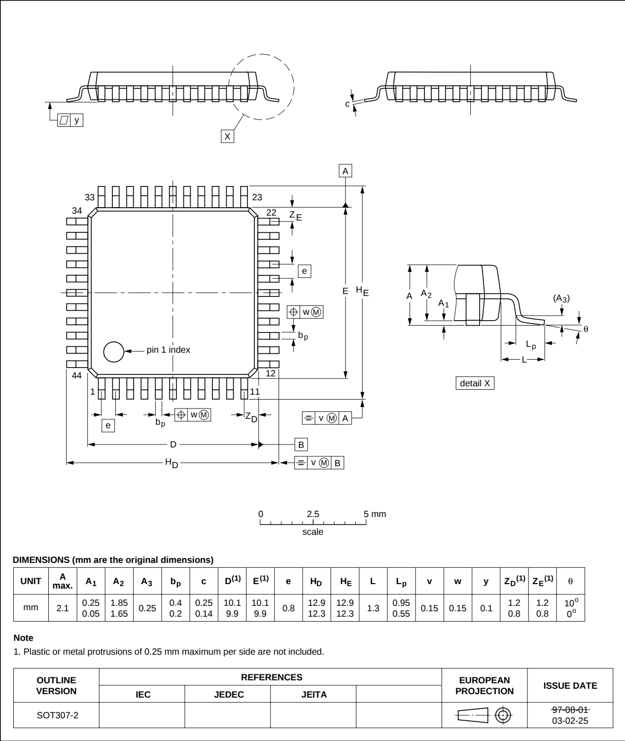
Fig 28. SOT307-2 (QFP44)
