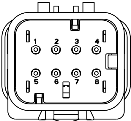
776538-2 SCALE 2:1
