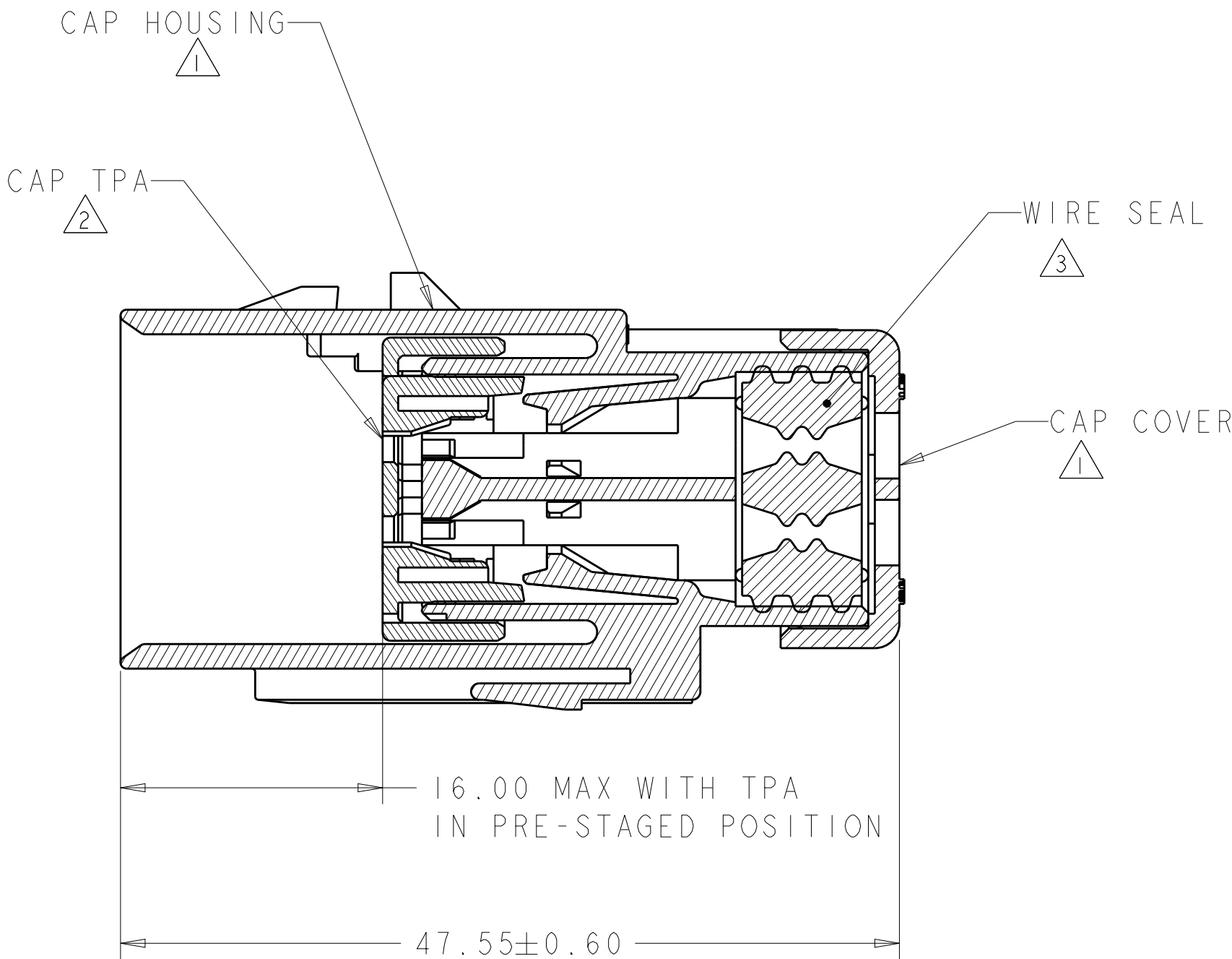
SECTION A-A
