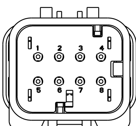
776538-4 SCALE 2:1
