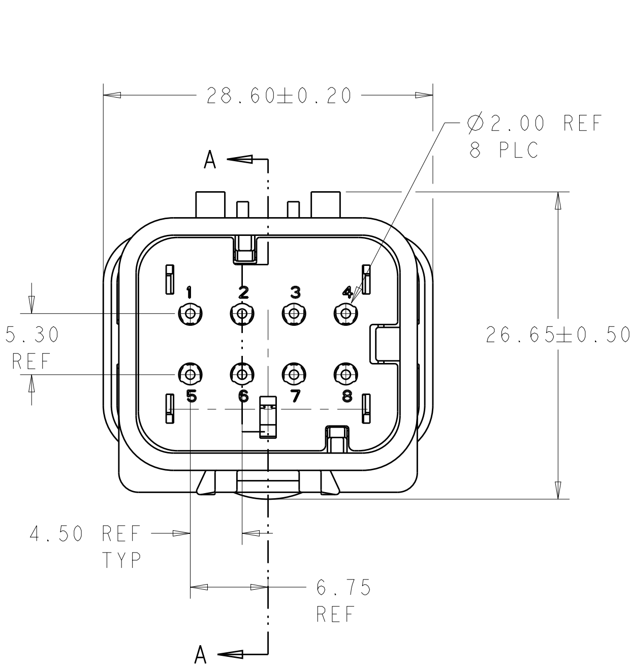
776538-1 SHOWN
