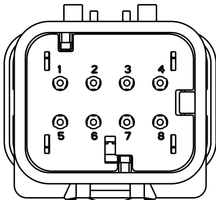
776538-3 SCALE 2:1
