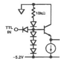
TTL Input Buffer
