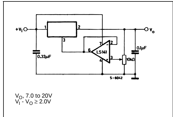
Figure 6 : DC Parameter
