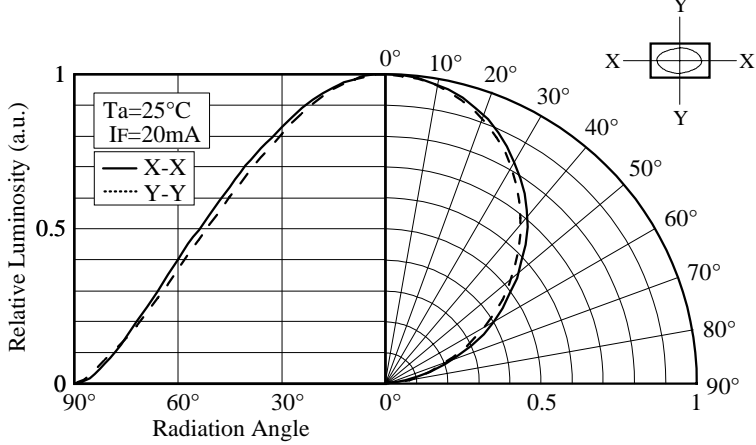
■ Directivity (NSCW335)
