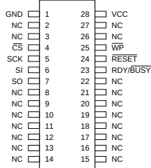
SOIC
