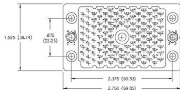
120 PIN RECEPTACLE
