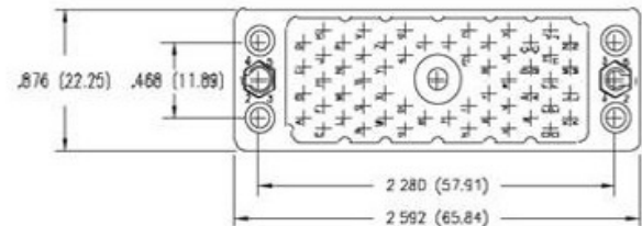
90 PIN RECEPTACLE
