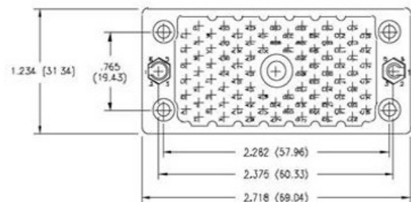
120 PIN RECEPTACLE
