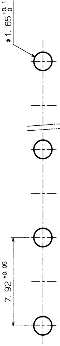
プリント基板穴明け寸法
