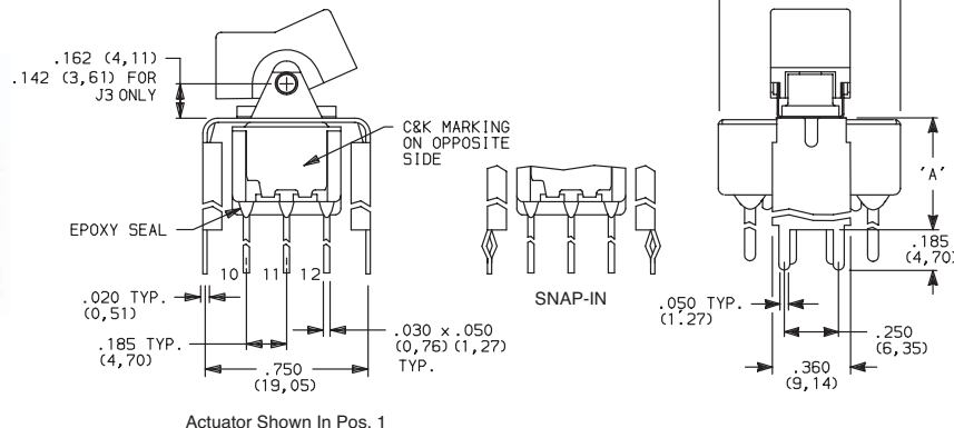
7401J1_BE2 4PDT
