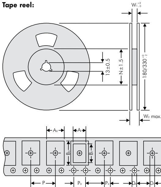
Tape reel:
