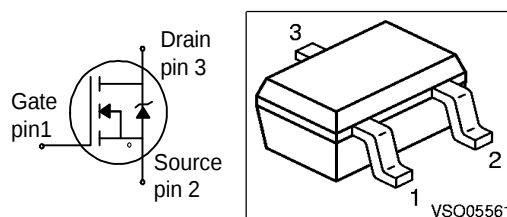
PG-SOT-323
