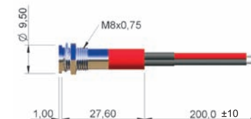
WIRES
