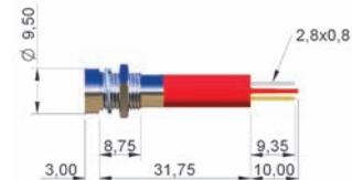
SOLDER LUG/FASTONS
