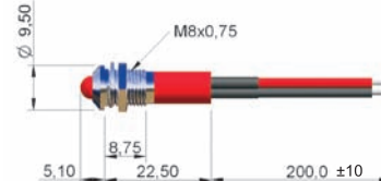
WIRES
