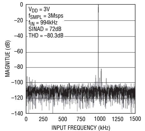
1MHz Sine Wave 8192 FFT Plot
