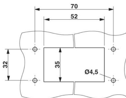
Montageausschnitt
