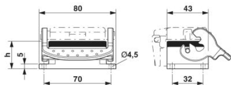
Maßzeichnung
