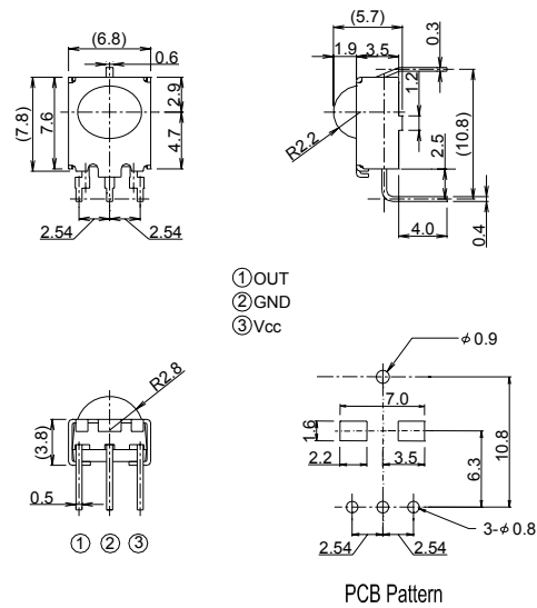
NJL31H000A-M UNIT:mm
