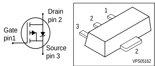
PG-SOT89
