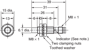
Fig. 29: E2E-X4MD□-M3G/E2E-X2ME□-M3/F□-M3
