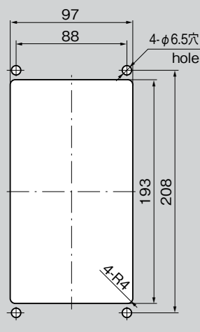
パネル穴明け寸法 Panel drilling dimensions
