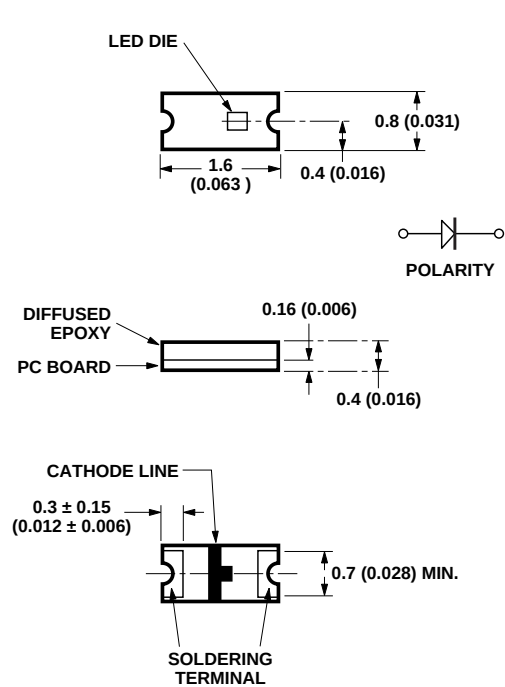
HSMW-B197
