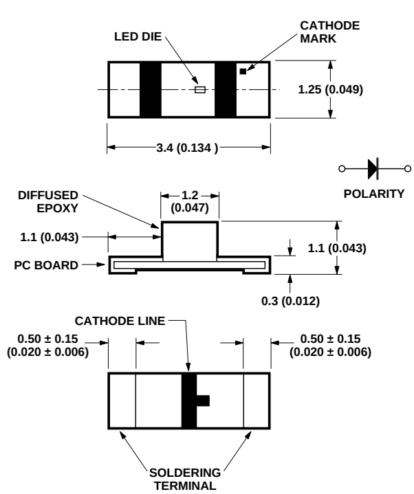
HSMW-B265
