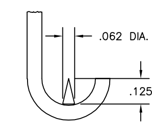
EXTENDED HOOK DETAIL 4X ACTUAL SIZE
