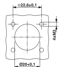
Einbaumaße: RF-1.S..8AAAK00 , RF-1.P..8AAAK00
