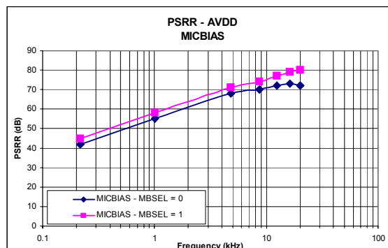
AVDD – MICBIAS
