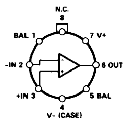
TO-99 (J-Suffix)
