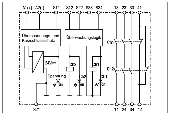
FIG. 38: RELAIS-BLOCKSCHALTBIld
