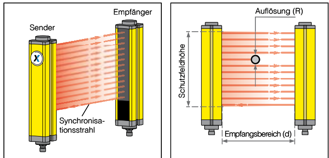
FIG. 18 + 19: FUNKTIONSPRINZIP
