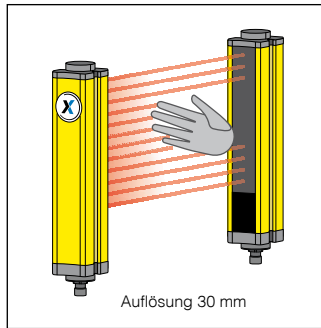
FIG. 1, 2 + 3: SCHUTZFELDAUFLÖSUNG
