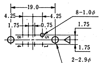
PD-1608
