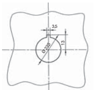
Bohrplan
