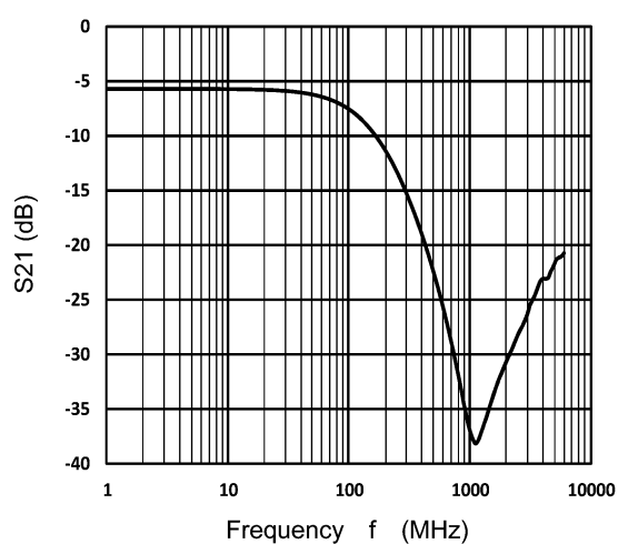
Fig. 10.1 S_{21} - f
