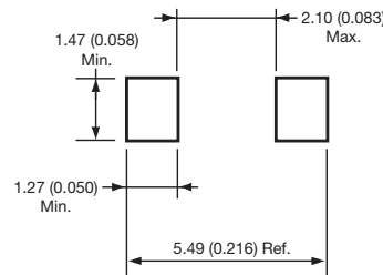
DO-214AC (SMA)
