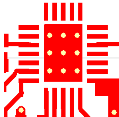
TOP (24 LD QFN)
