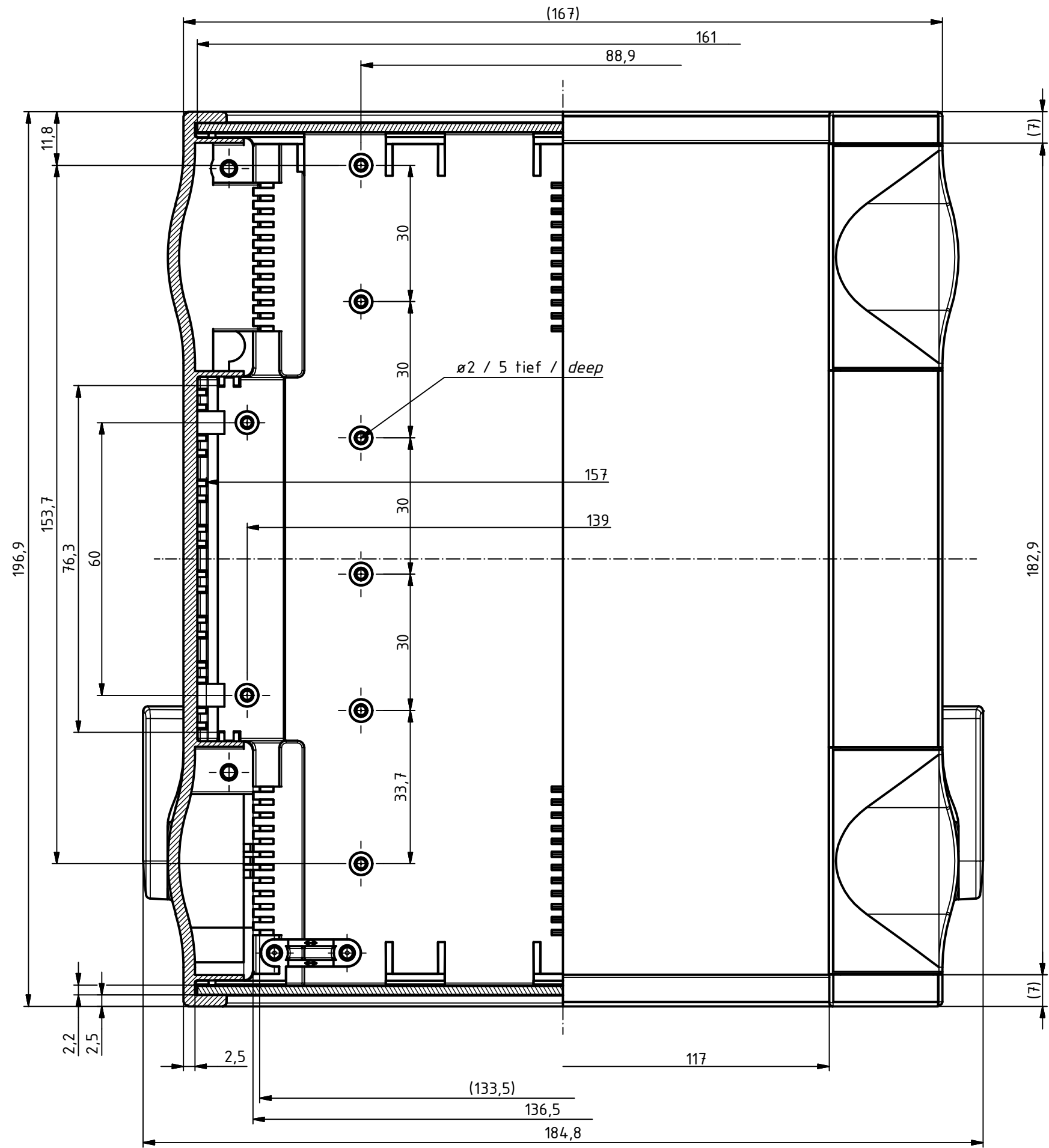
B-B ( 1 : 1 )
