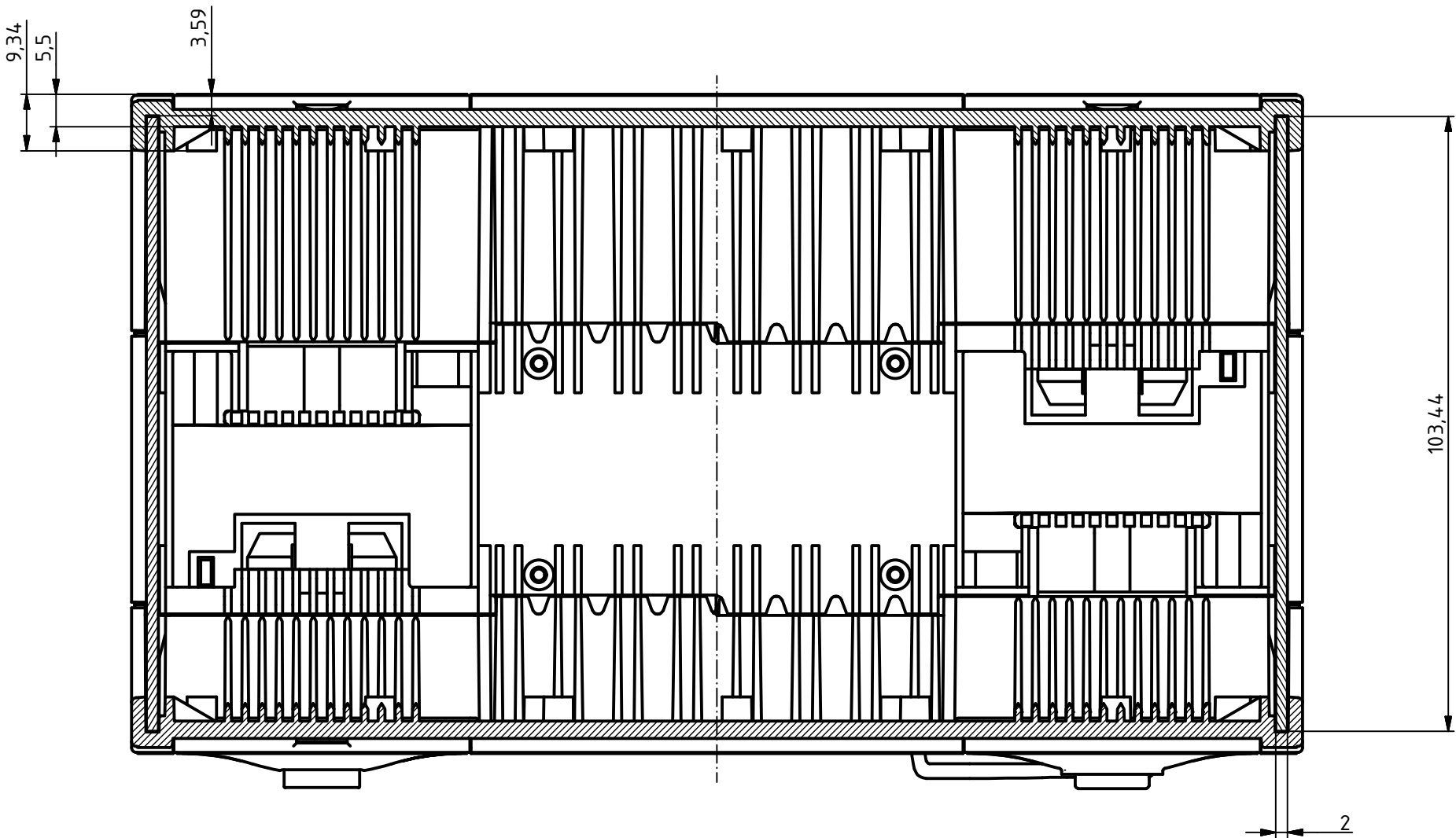
A-A ( 1 : 1 )
