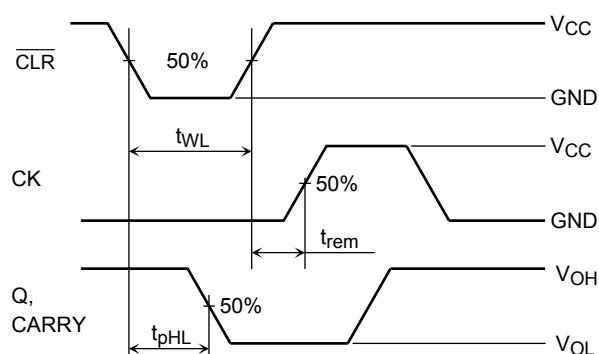
クリアモード (TC74AC163)
