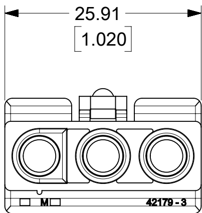
3 CIRCUIT RECEPTACLE
