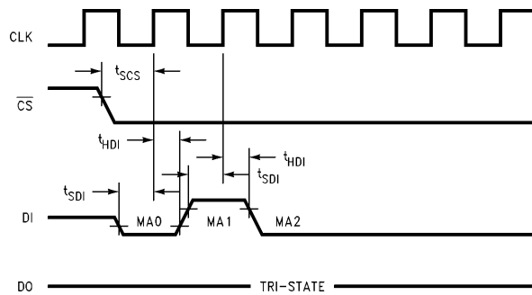
FIGURE 2. DI Timing
