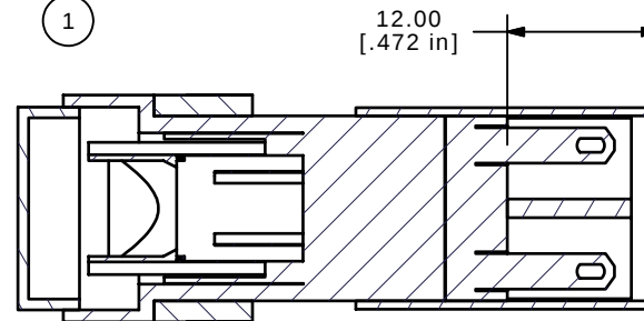
SECTION A-A SCALE 1.50 : 1
