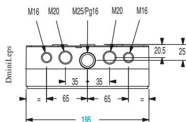
8 modules
