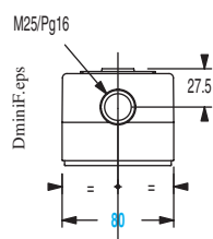
3 modules
